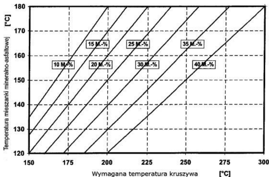
Tablica 13. Temperatura kruszywa w zależności od ilości zimnego i suchego
