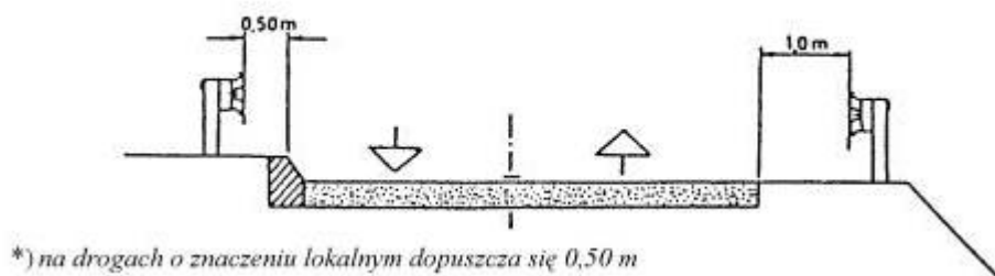
Załącznik 11.6. Sposoby lokalizowania barier w przekroju poprzecznym drogi, wg [32]
